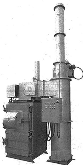
廃プラ対応焼却炉「ISRRモデル」
