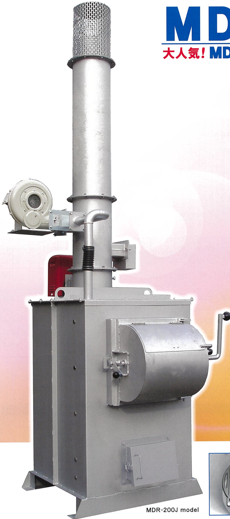
▲ロストル装備
