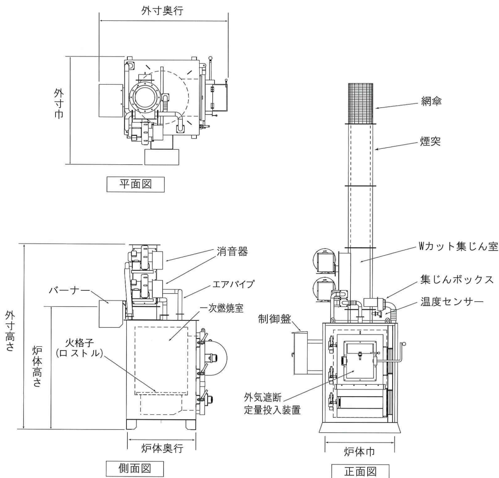
図面はSPR-500J
