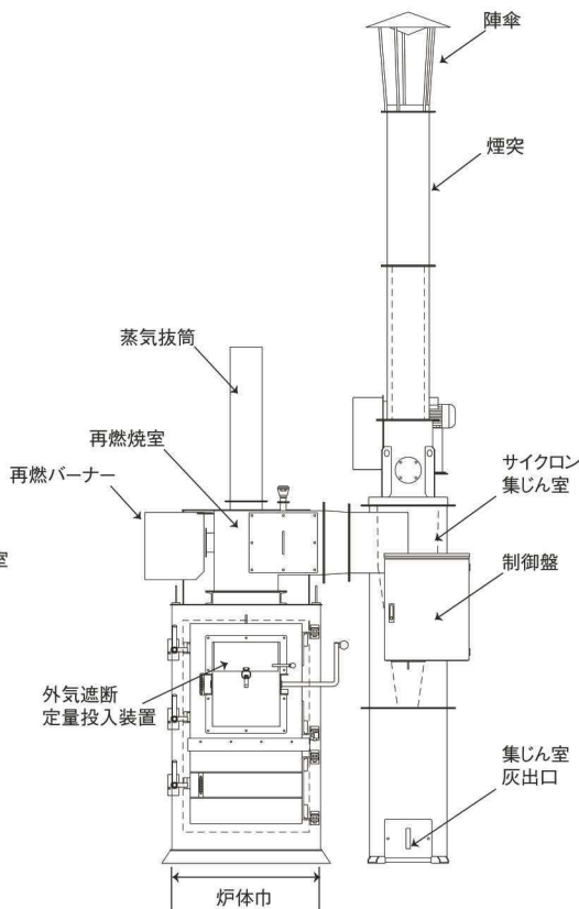
正面図
