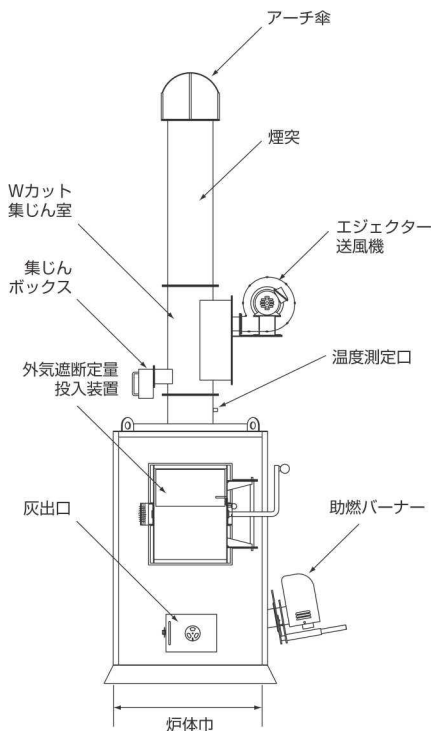
正面図
