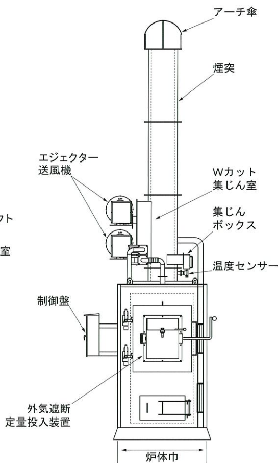
正面図
