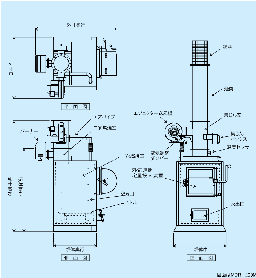
図面はMDR-200M
